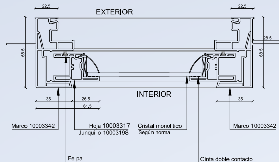
Detalle 2
