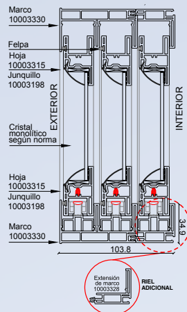
Detalle 2
