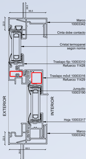
Detalle 1
