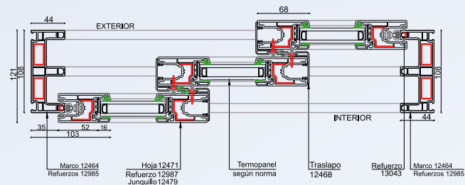
Detalle 2
