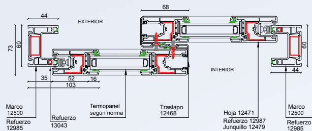
Detalle 2
